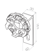
23 615.9101 gekröpft, bis max. 50 Nm (60 mm Wandabstand)
