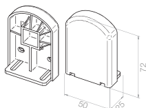
Antriebslager
