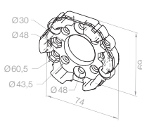
23 003.0001 Teilkreis 48/Teilkreis 60 (Alu)
