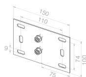
24 554.0001 für Universallager (23 004.0001 und 23 615.4401)
