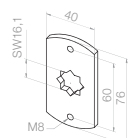
13 103.4001 Teilkreis 60 mm, flach
