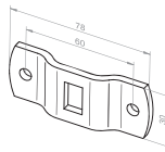
13 106.1701 Wandanker gekröpft, Teilkreis 60 mm
