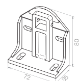
Lagerbock
