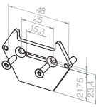
23 374.7301 Adapterplatte mit Schlitz 3 x 15 mm
