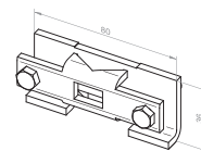
23 965.0003 Klemmlager für Rollenlagerhalter oder für Eingipswandanker
