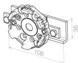
23 615.7201 für Rollenlagerhalter Drehmomentbegrenzung bis max. 30 Nm
