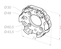
23 003.0301 Teilkreis 48/Teilkreis 60 mit Gewinde M6/M8 – für Markisen –
