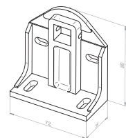
13 109.1701 Lagerbock Motorseite bis 20 Nm
