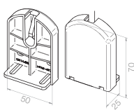
Achsträgerlager
