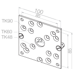
23 687.0501 mit 2 versenkbaren Schrauben M6 x 16 und Muttern
