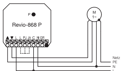
Anschluss Antrieb
