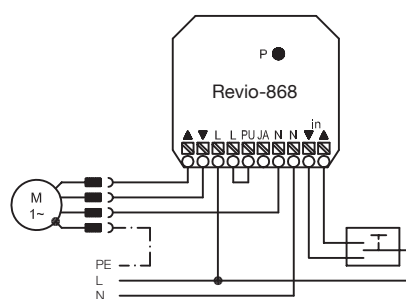
Jalousie im Pulse-Betrieb
