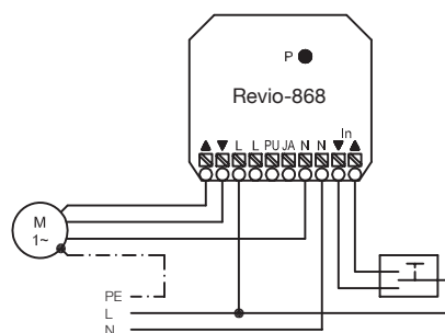
Anschluss Rohrmotor
