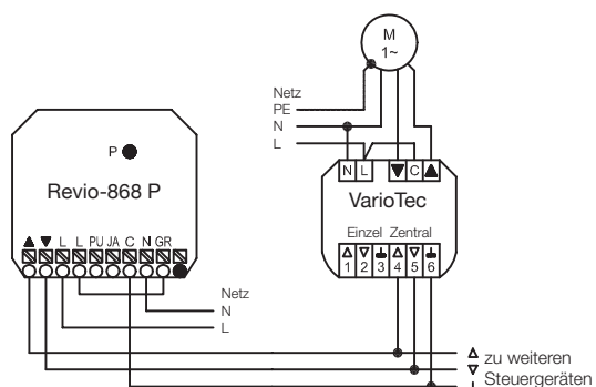
Anschluss ProLine-Steuergerät
