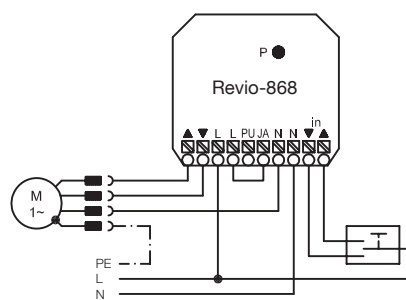
Anschluss Jalousiemotor
