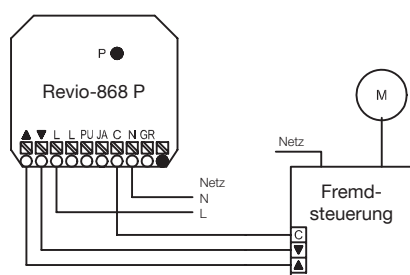
Anschluss Antrieb und Fremdsteuerung
