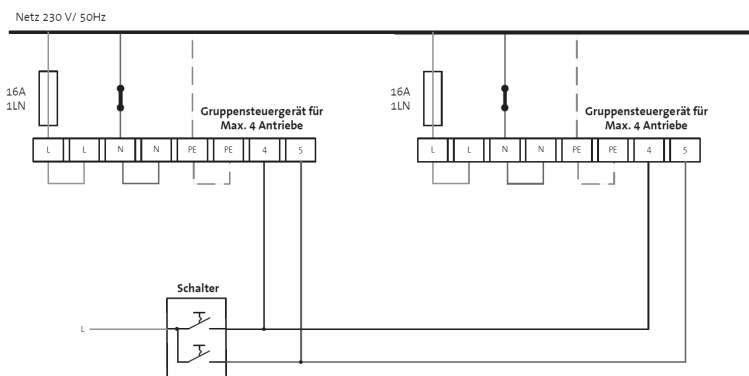
Anschlussbeispiel mit 2 Gruppensteuergeräte parallel geschaltet
